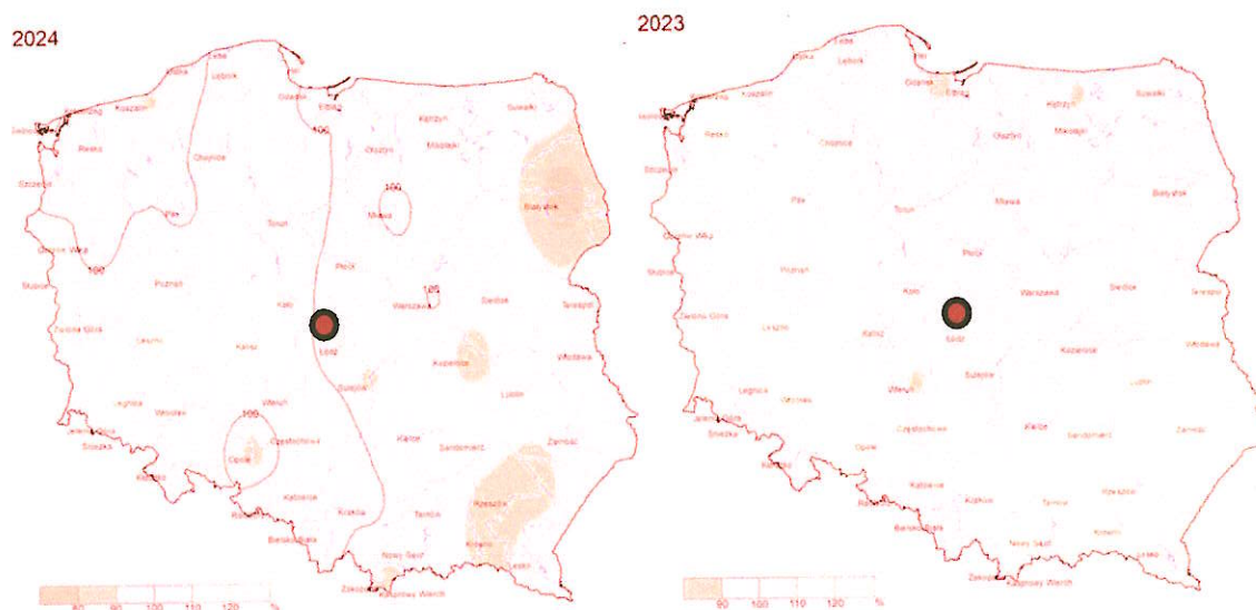
Rysunek 6 Anomalie sumy opadów w Polsce w latach 2023-2025 r.
