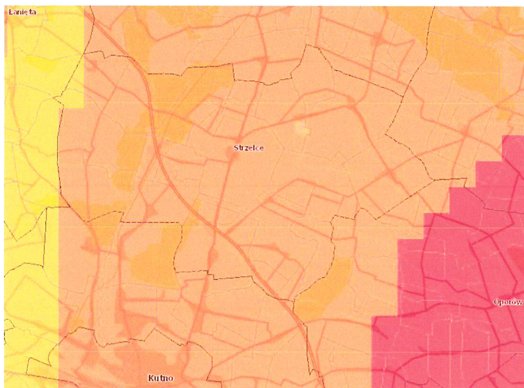
Rysunek 11 Mapa zagrożenia suszą atmosferyczną
