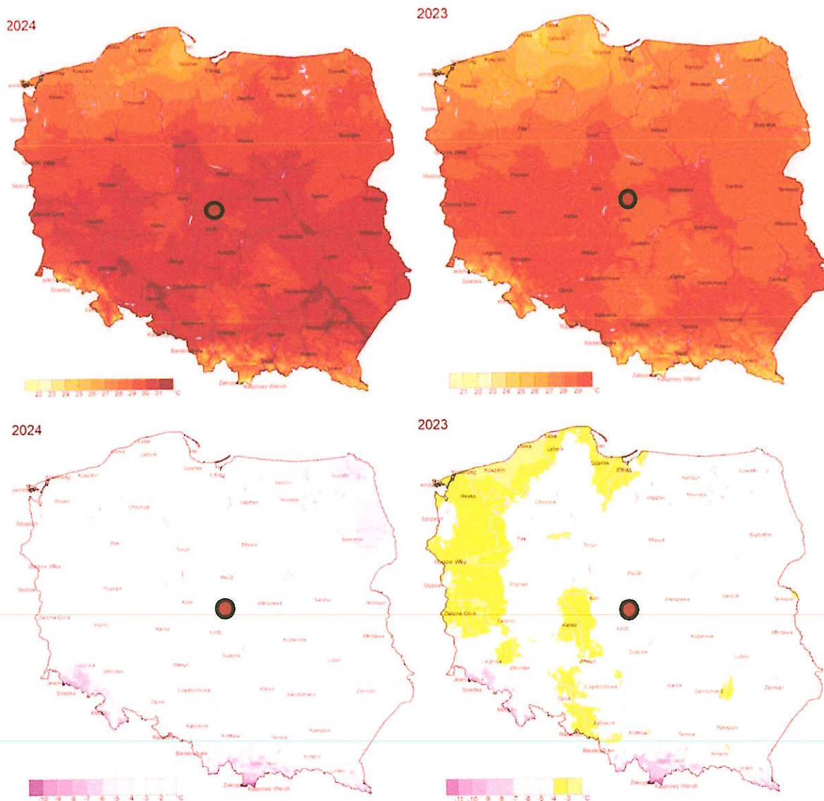
Rysunek 5 Ekstremalne temperatury maksymalne i minimalne w Polsce w latach 2023-2024
